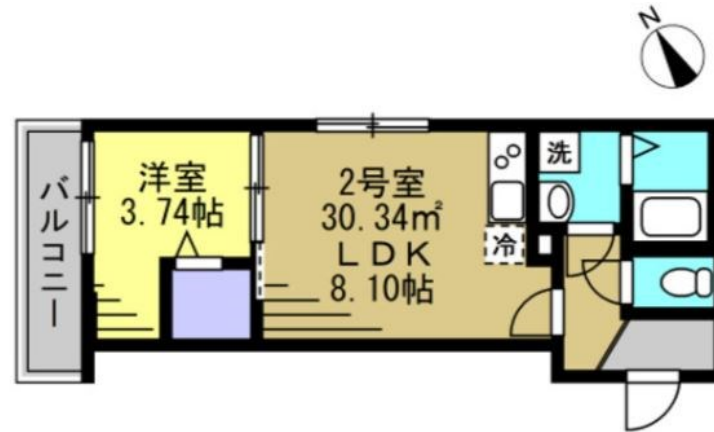
【間取り図】
